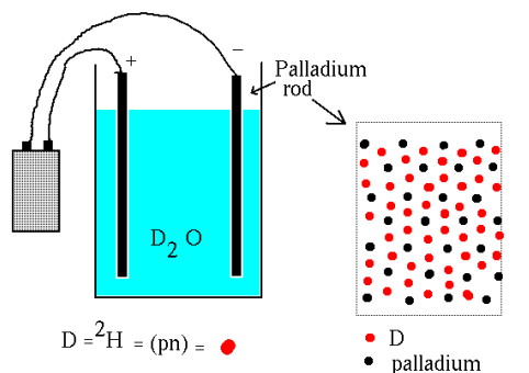
圖：cold fusion
