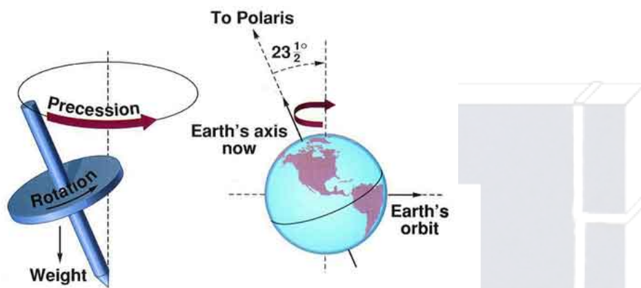
圖：precession
